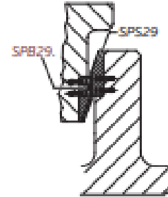
Montaj Örneği Mounting example
