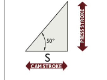
Kam Diyagramı / Cam Diagram
