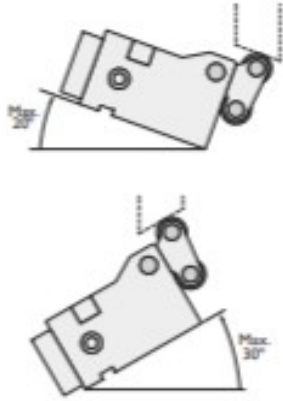
Çalışma Açısı / Work Angle
