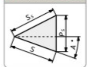
Kam Diyagramı / Cam Diagram
