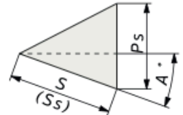
■ Kam Diyagramı / Cam Diagram
